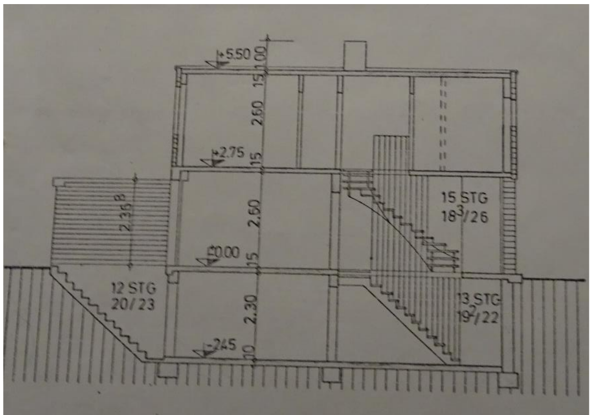
Schnitt
